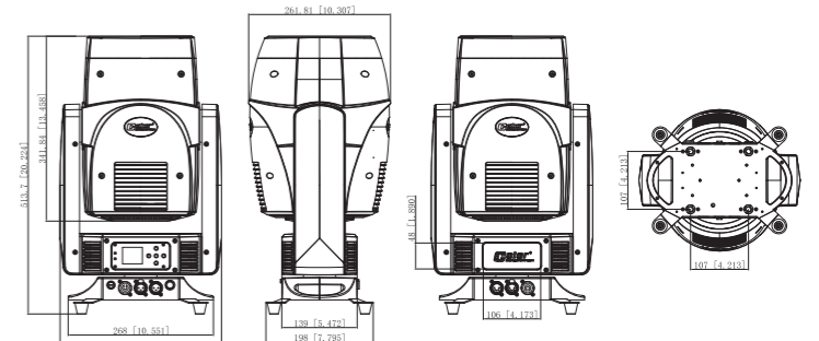
尺寸图
