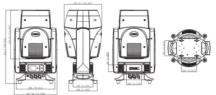
尺寸图
