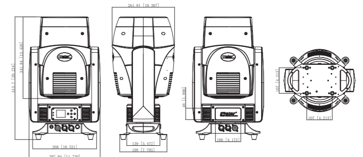
尺寸图
